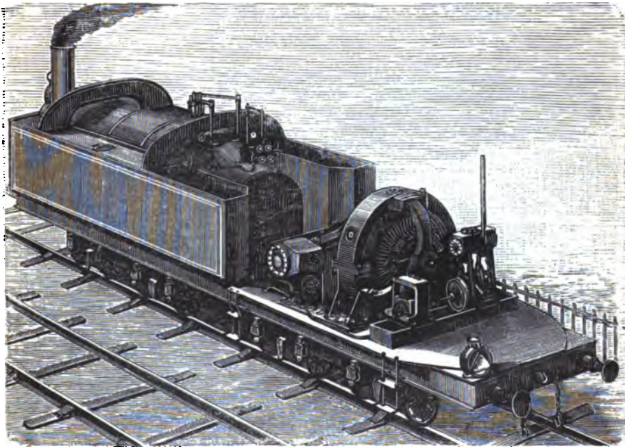
2. Электрическій локомотивъ Гейльмана (при снятой будкѣ).
